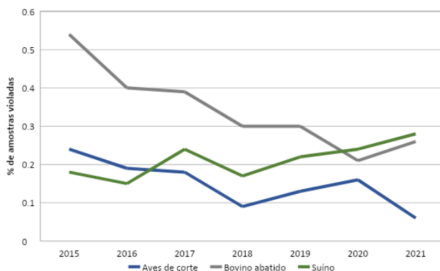
Figura 14. Frequência de violação (% de amostras violadas) do Subprograma de Monitoramento do PNCRC de bovinos, aves e suínos abatidos, Brasil, 2015 a 2021.
