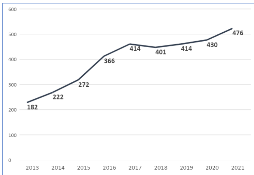
Figura 11. Número de substâncias testadas (analisadas) no Plano Nacional de Controle de Resíduos e Contaminantes – PNCRC Animal, Brasil, 2013 a 2021.
