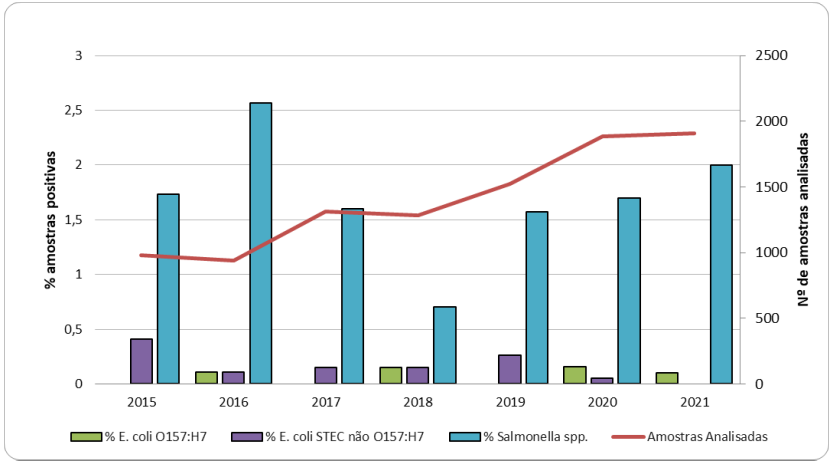
Figura 3. Número de amostras analisadas e percentual de amostras positivas nas amostras coletadas para verificação oficial de E. coli STEC e Salmonella spp. em carne de bovinos, Serviço de Inspeção Federal, Brasil, 2015 a 2021.
