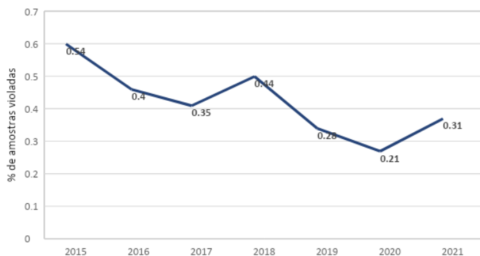
Figura 13. Frequência geral de violação (% de amostras violadas) observada no Subprograma de Monitoramento do PNCRC Animal (todas espécies e produtos monitorados), Brasil, 2015 a 2021
