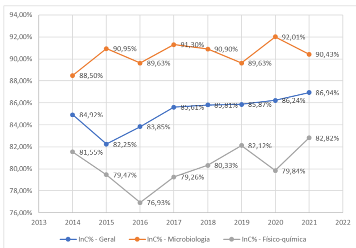
Figura 6. Índice de conformidade percentual (InC %) das amostras de produtos de origem animal geral, para parâmetros microbiológicos e para parâmetros físico-químicos, Serviço de Inspeção Federal, Brasil, 2014 a 2021.
