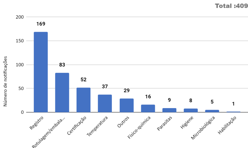
Figura 10. Número de notificações de irregularidades não passíveis de RAI, Brasil, 2021.
