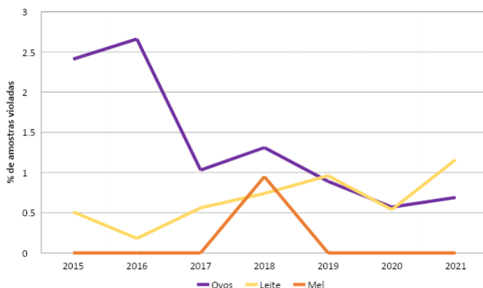
Figura 15. Frequência de violação (% de amostras violadas) do Subprograma de Monitoramento do PNCRC de leite, ovos e mel, Brasil, 2015 a 2021.
