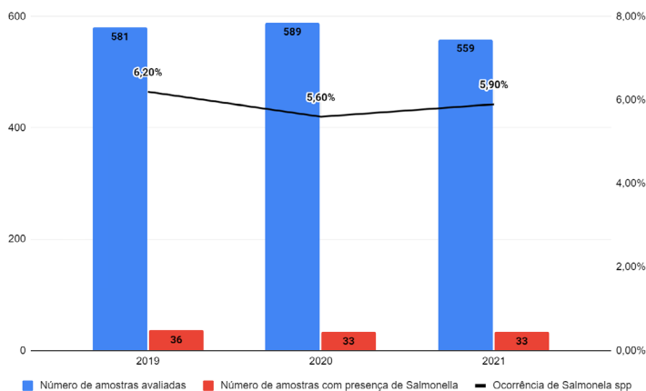
Figura 4. Ocorrência de Salmonella spp. em amostras oficiais de esfregaço de superfície de carcaça de suínos, Serviço de Inspeção Federal, Brasil, 2019 - 2021.
