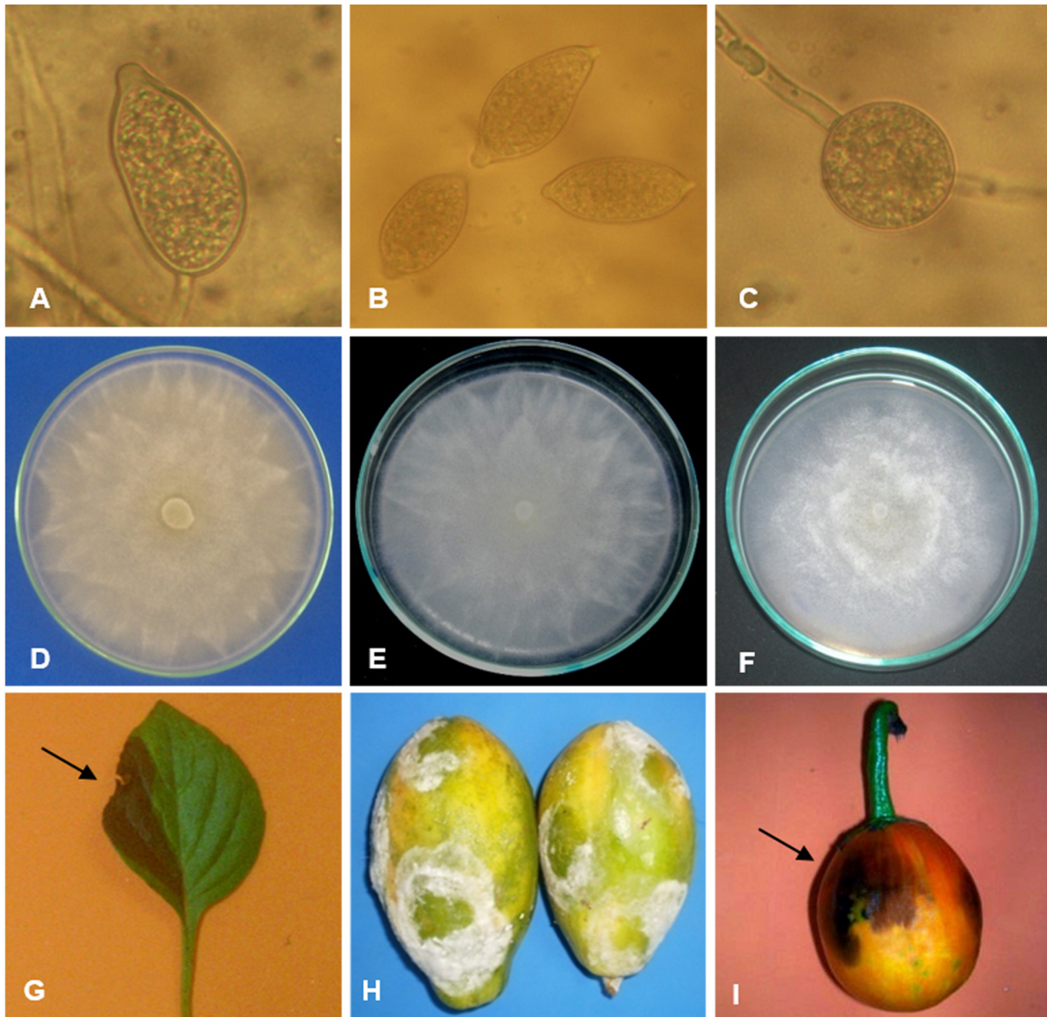
Figura 1 - Caracterização dos isolados de Phytophthora palmivora do Sul da Bahia quanto a morfologia, fisiologia e patogenicidade. Estruturas assexuadas dos isolados: esporângios, 1333 (A) e 1108 (B); clamidósporo, 1329 (C). Tipo de colônias dos isolados em meio de cultura cenoura-água, aos sete dias de idade: crisântemo - 1329 (D) e 1107 (E); concêntrica - 1108 (F). Lesões causadas, em testes in vitro , por isolados em folha de manjeriço (seta) - 1107 (G), em frutos de mamoeiro - 1189 (H) e em fruto de jiló (seta) - 1333 (I).
