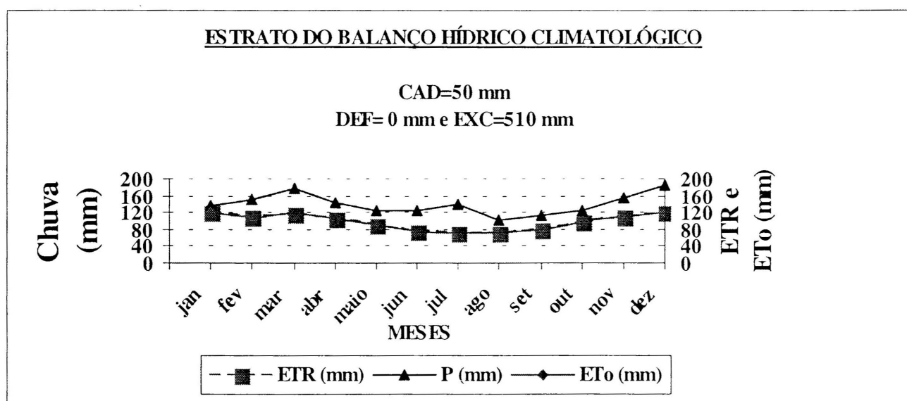
Figura 3. Estrato do balanço hídrico climatológico mensal (média do período) para a área de abrangência do município de Ilhéus, BA, e para uma capacidade máxima de armazenamento de água no solo de 50 mm.
