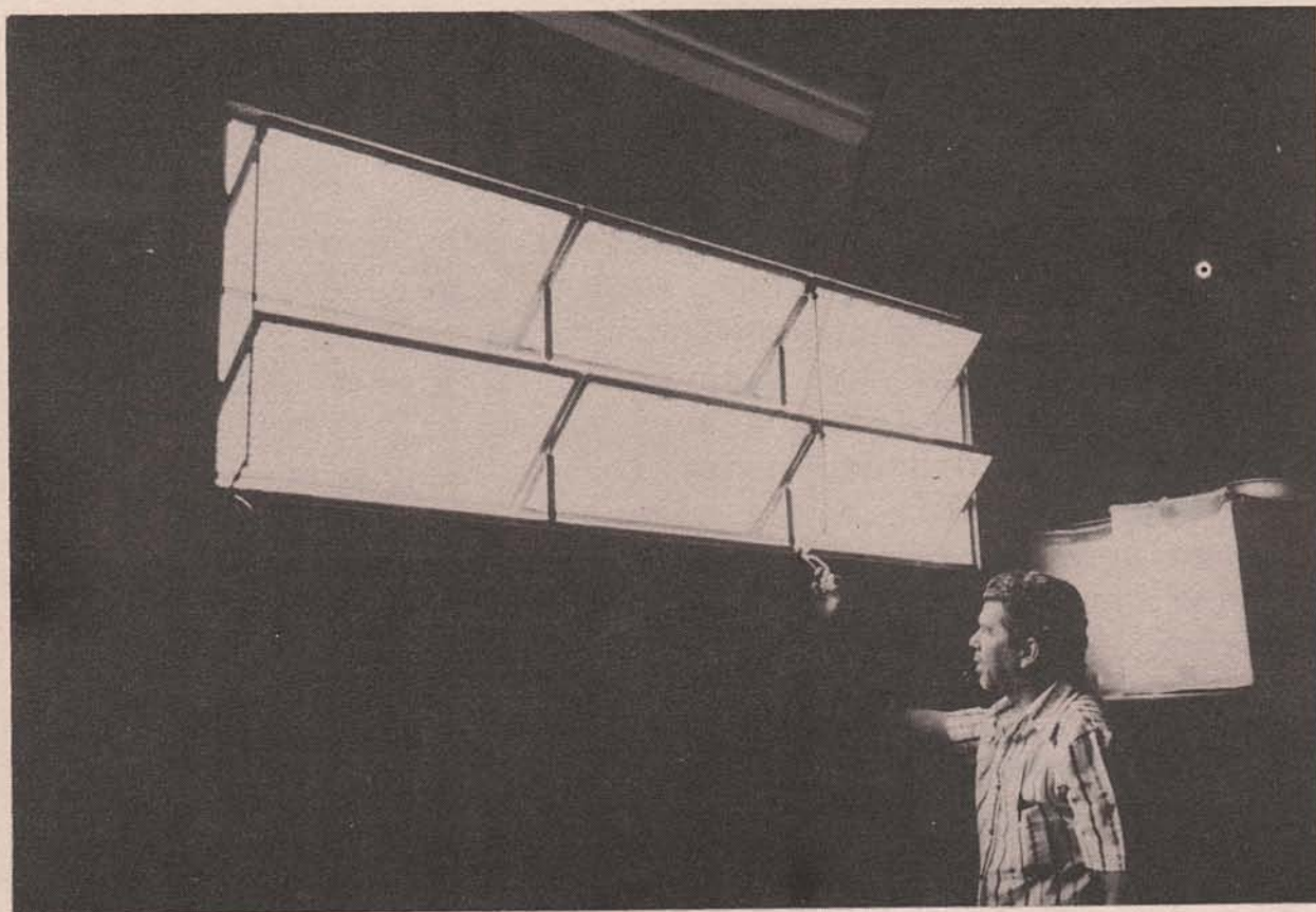
Figura 5 — Sistema de controle manual de ventilação em armazém de cacau.
