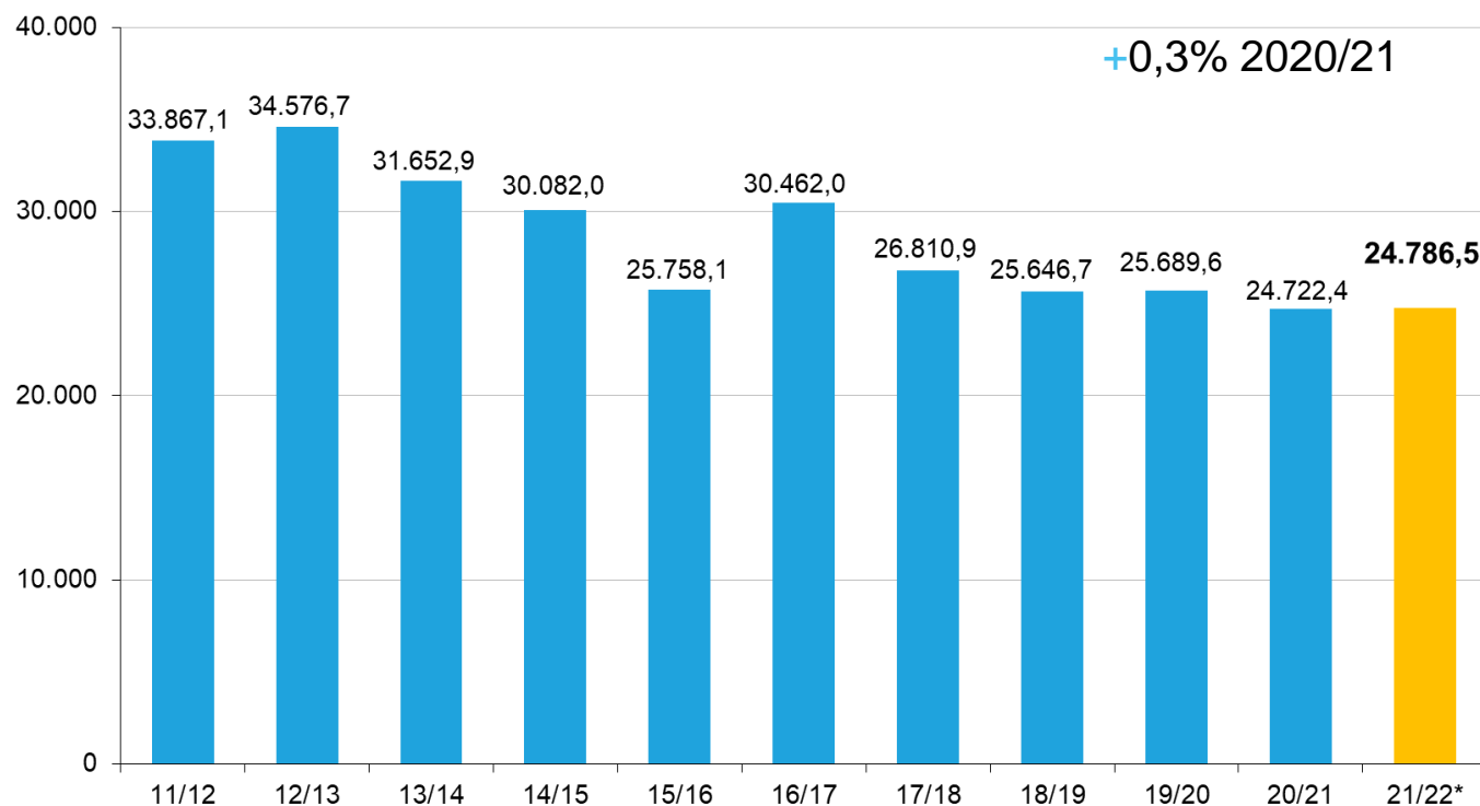
PRODUTIVIDADE (kg/ha)
