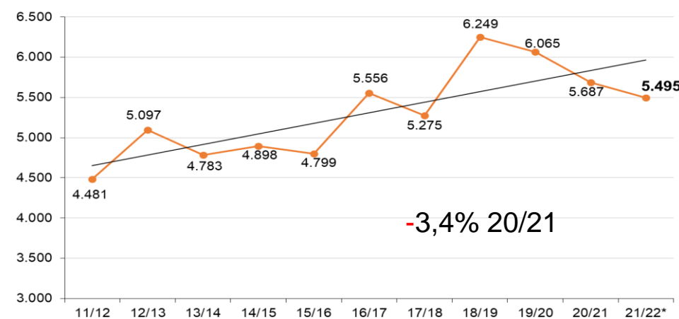
PRODUTIVIDADE (kg/ha)
