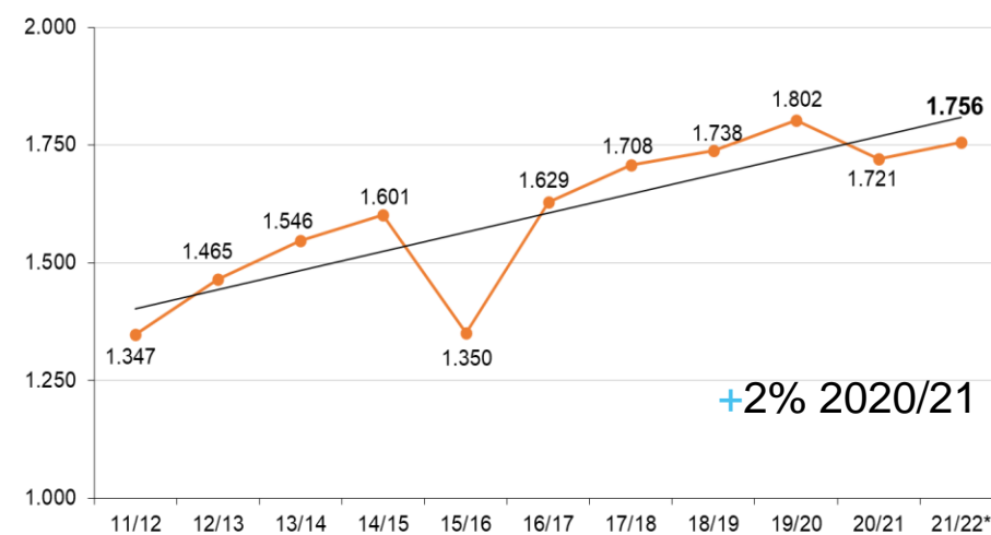
PRODUTIVIDADE (kg/ha)
