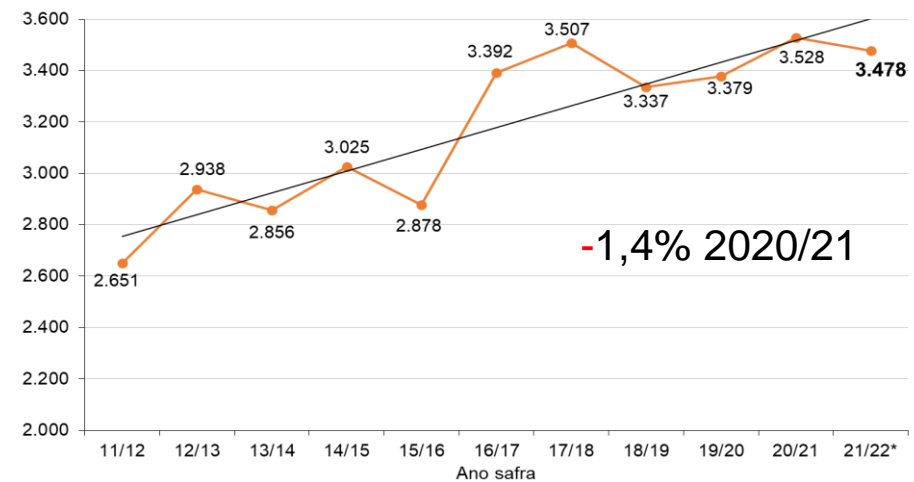
PRODUTIVIDADE (kg/ha)
