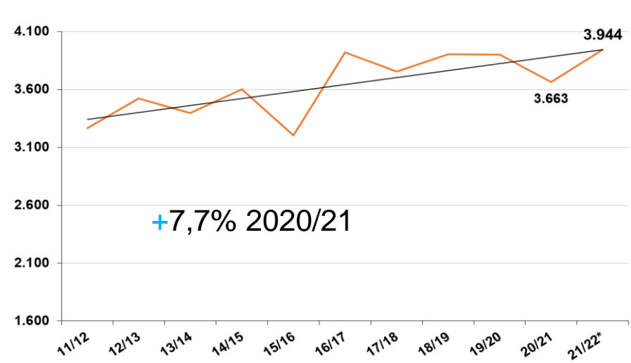
PRODUTIVIDADE (kg/ha)
