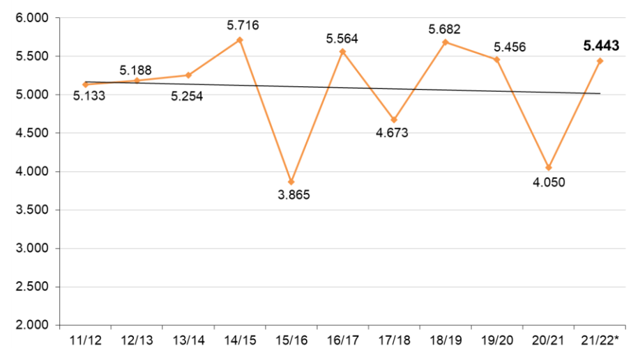
PRODUTIVIDADE (kg/ha)
