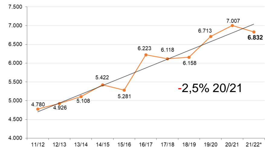
PRODUTIVIDADE (kg/ha)
