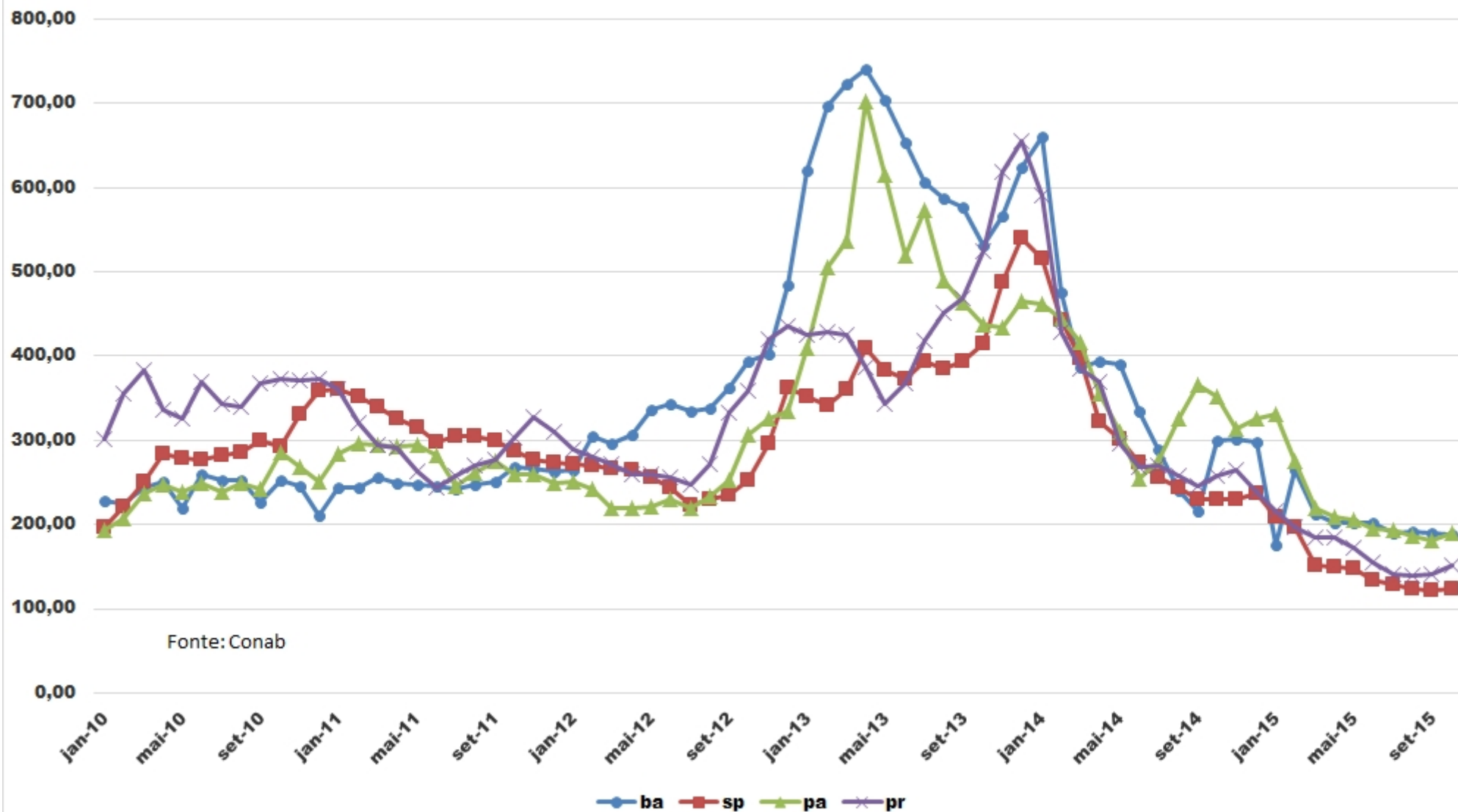
Gráfico 2: Evolução dos preços reais recebidos pelos produtores de raiz de mandioca (R$/t) - jan/10-out/15
