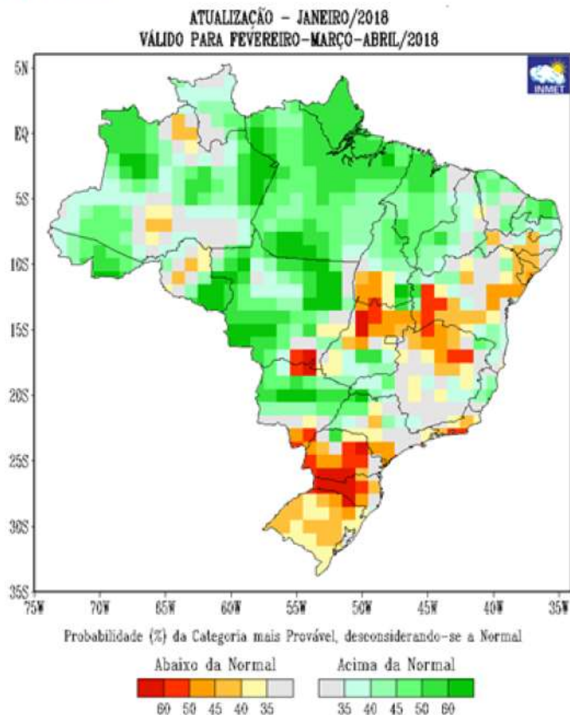
Figura 4 - Previsão probabilística de precipitação do modelo estatístico do INMET para o trimestre FMA/2018
