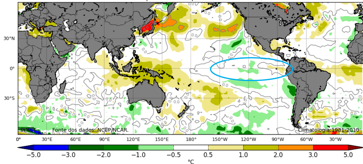
Anomalia da Temperatura da Superfície do Mar - 01-15/08/2021
