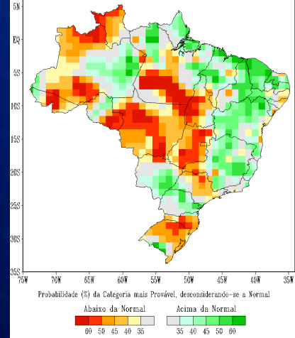
PREVISÃO PROBABILÍSTICA EM TERCEIS - PRECIPITAÇÃO ATUALIZAÇÃO - AGOSTO/2021 VÁLIDO PARA OUTUBRO/2021
