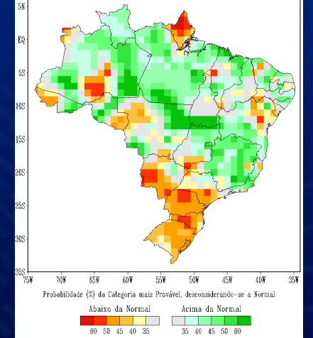
PREVISÃO PROBABILÍSTICA EM TERCEIS - PRECIPITAÇÃO ATUALIZAÇÃO - AGOSTO/2021 VÁLIDO PARA NOVEMBRO/2021
