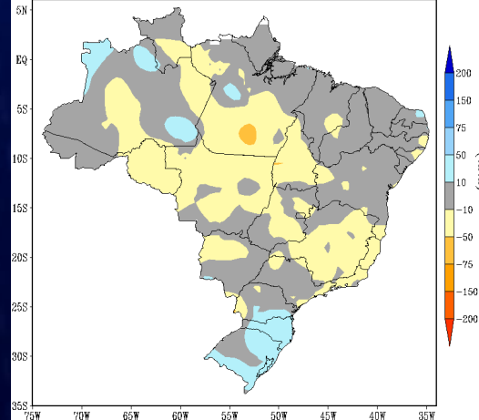
PREVISÃO DE ANOMALIAS DE PRECIPITAÇÃO (mm) ATUALIZAÇÃO - AGOSTO/2021 VÁLIDO PARA SETEMBRO/2021
