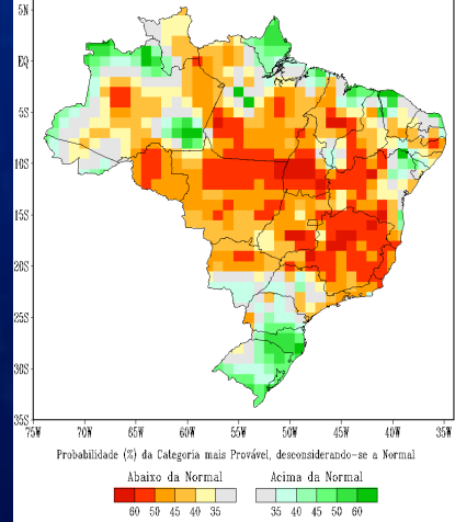
PREVISÃO PROBABILÍSTICA EM TERCEIS - PRECIPITAÇÃO ATUALIZAÇÃO - AGOSTO/2021 VÁLIDO PARA SETEMBRO/2021
