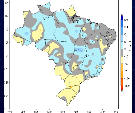
PREVISÃO DE ANOMALIAS DE PRECIPITAÇÃO (mm) ATUALIZAÇÃO - AGOSTO/2021 VÁLIDO PARA NOVEMBRO/2021
