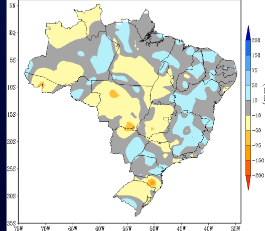
PREVISÃO DE ANOMALIAS DE PRECIPITAÇÃO (mm) ATUALIZAÇÃO - AGOSTO/2021 VÁLIDO PARA OUTUBRO/2021
