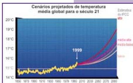
Figura 5.8. As estimativas analisadas pelo IPCC mostram que, no século 21, a temperatura média do planeta aumentará 1,8°C, em um cenário de baixas emissões, podendo chegar a 4°C no cenário de altas emissões.
