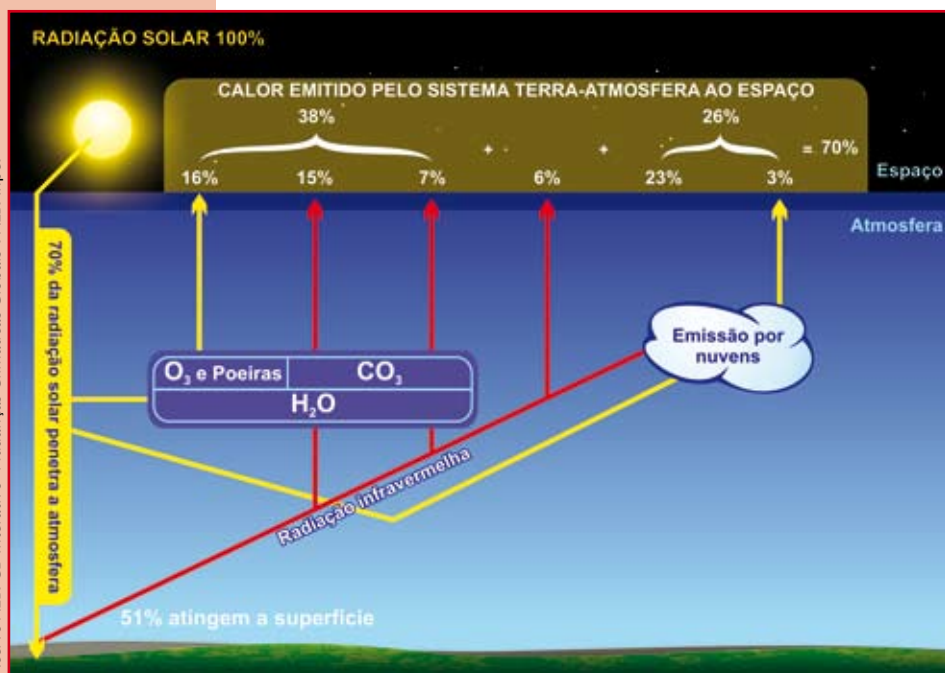
Figura 1.9. Balanço de Energia no Sistema Terra-Atmosfera.
