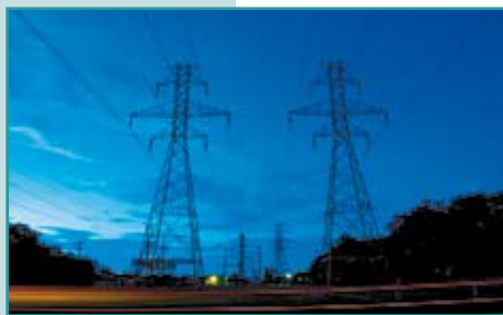
Figura 7.2. O setor de Energia, que responde por 65% das emissões de gases de efeito estufa, pode colaborar na redução dessas emissões se houver uma mudança sensível no padrão de investimento.
