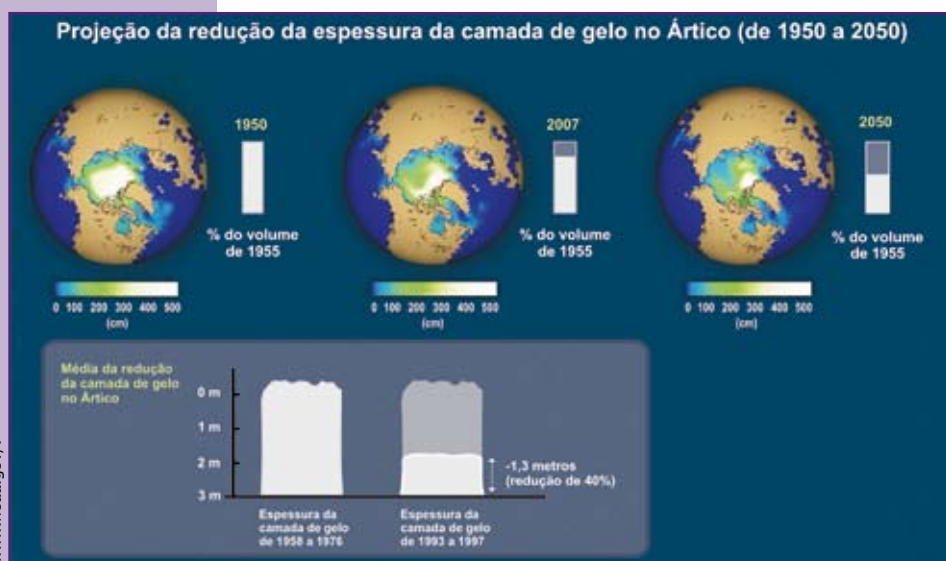
Figura 5.9. Os estudos indicam que a espessura do gelo no Ártico diminuiu 40% nas últimas décadas. A média de redução da espessura do gelo no Ártico, por década, é de 2,7%.
